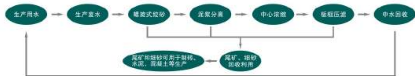
细砂、尾矿、中水回收利用示意图
